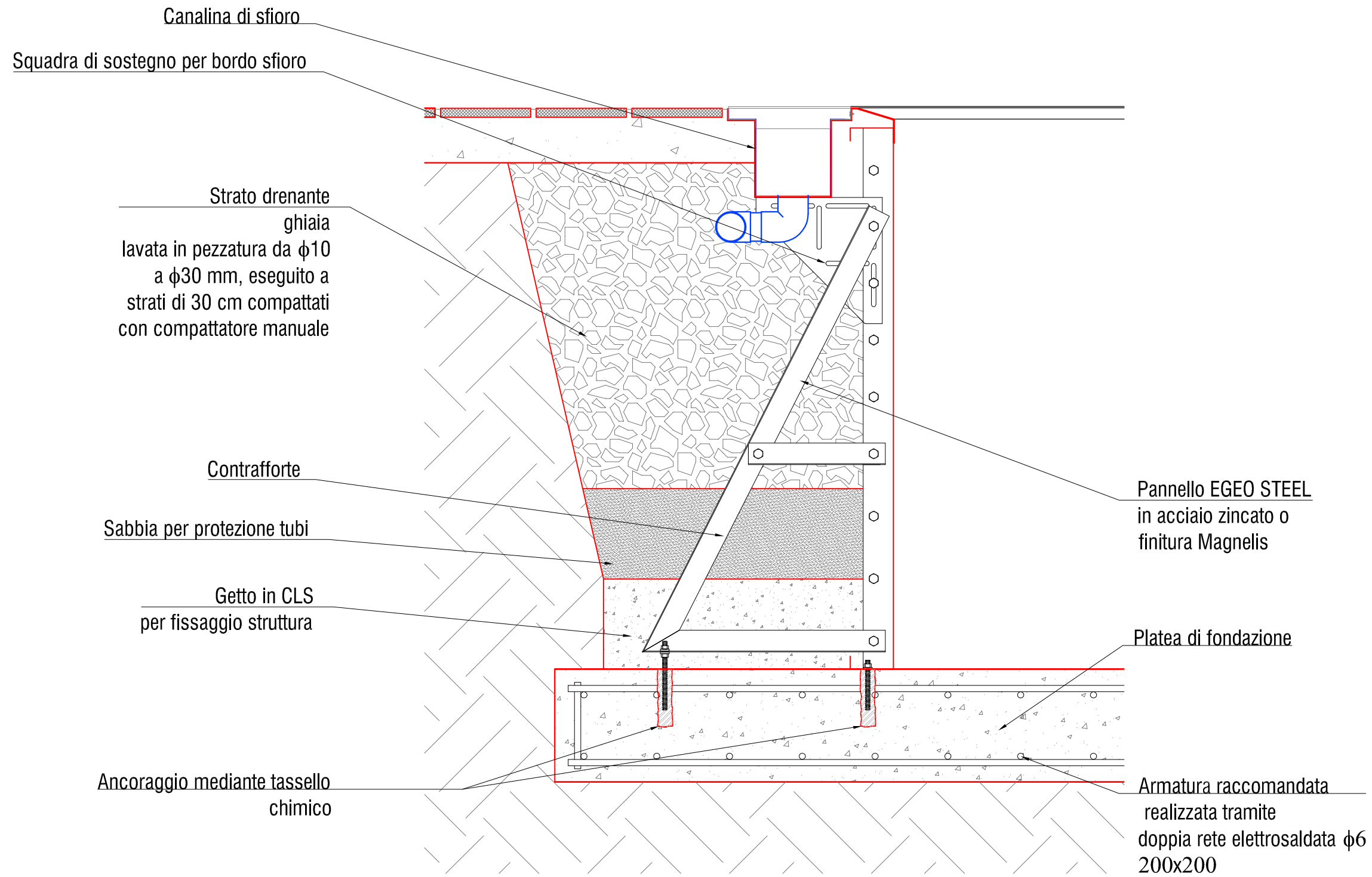
1 SEZIONE TIPO Scala: 1:10
