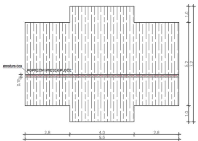
poprečni presek bazena 9,15x4,7 OSNOVA BAZENA
