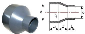
Konusna duga redukcija (lepak x lepak)
